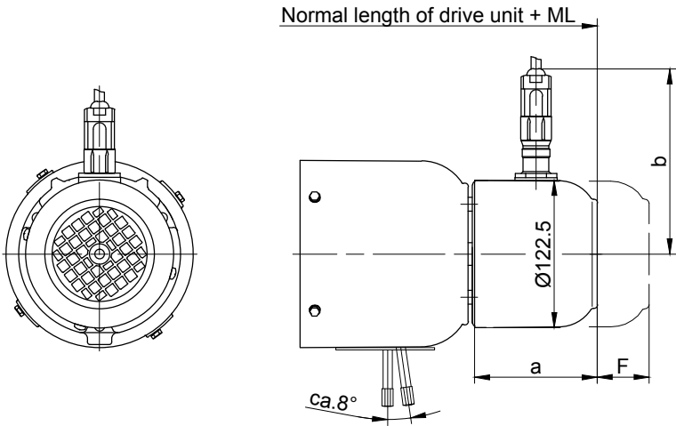
S..08-S..11
